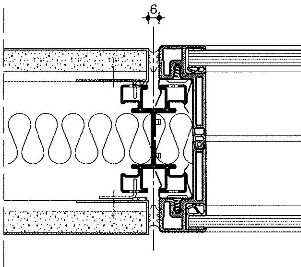
Vollbeplankung / Vollverglasung M 1:2
