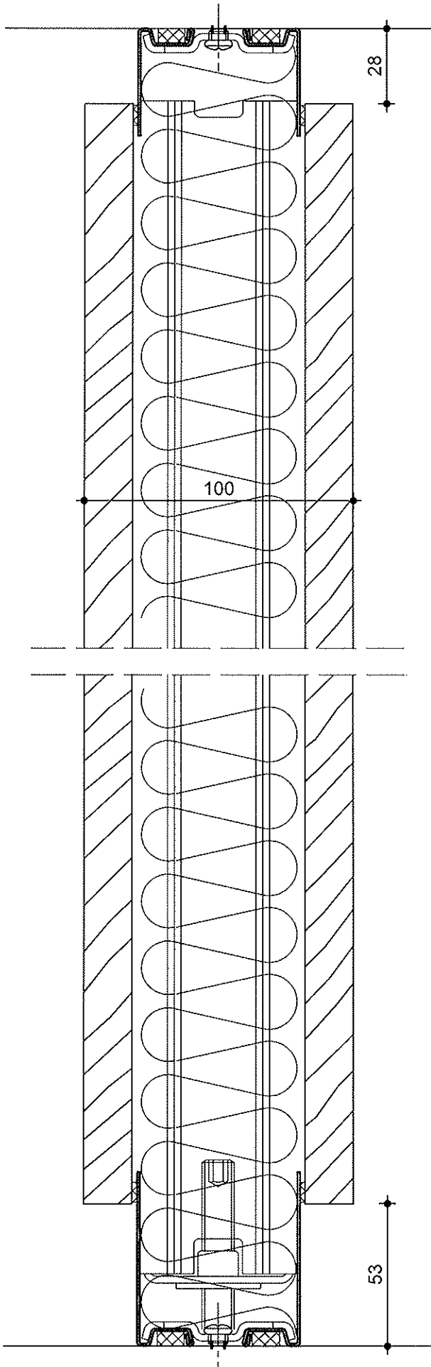
Vollbeplankung M 1:2
