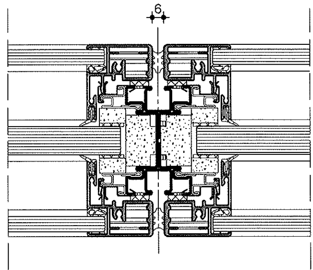
Vollverglasung EI30 M 1:2
