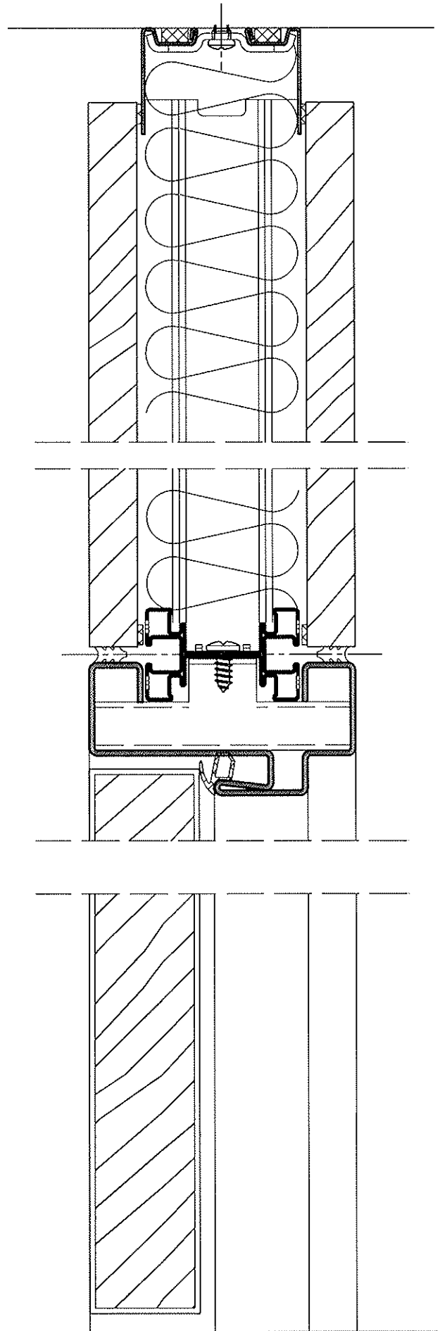
Türzarge M 1:2
