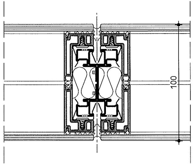
Vollverglasung M 1:2
