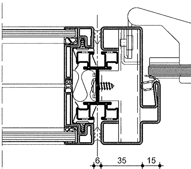
Vollverglasung / Türzarge M 1:2
