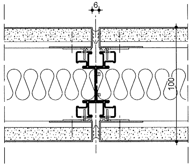
Vollbeplankung M 1:2
