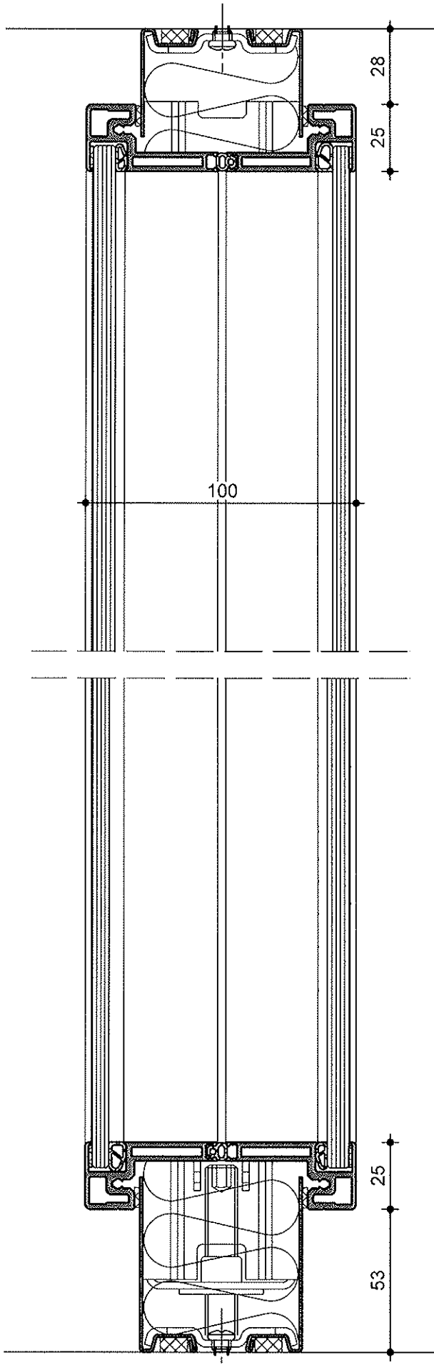
Verglasung M 1:2
