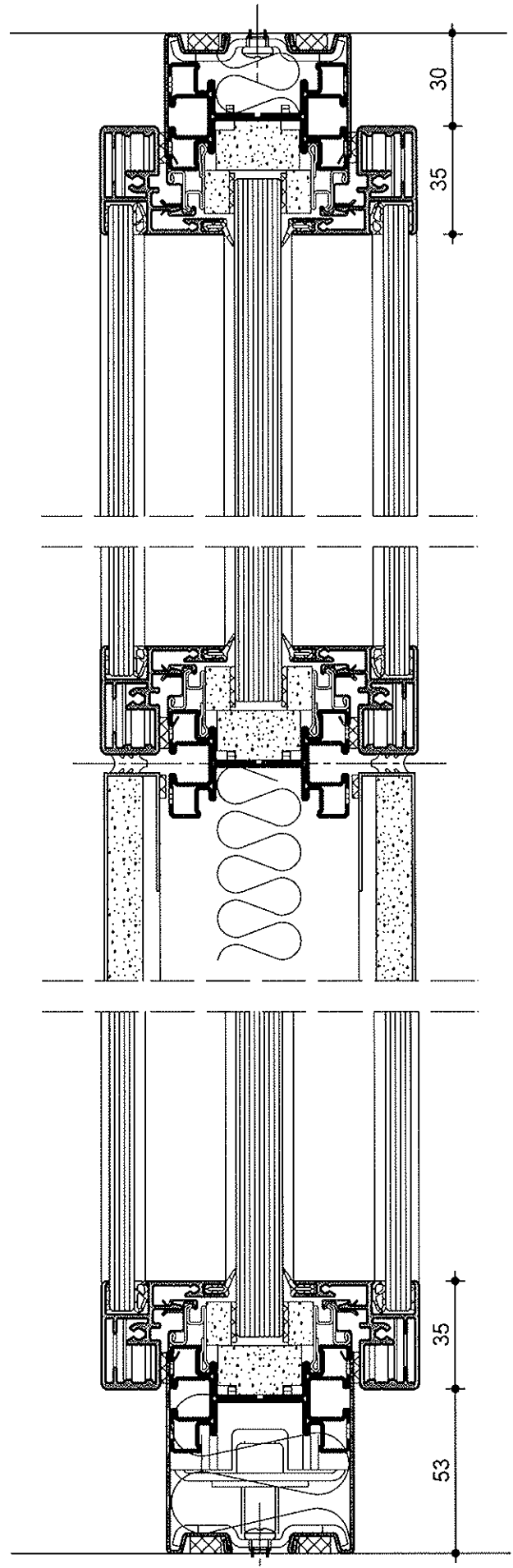
Verglasung EI30 M 1:2
