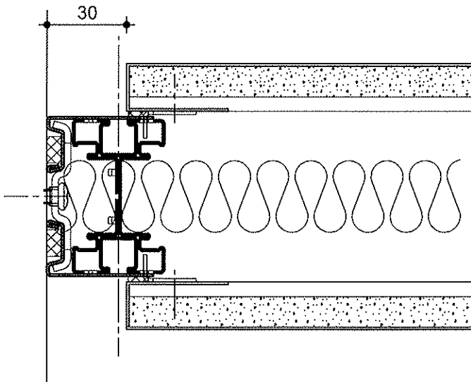
Wandanschluss M 1:2
