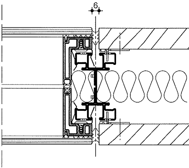
Vollverglasung / Vollbeplankung M 1:2
