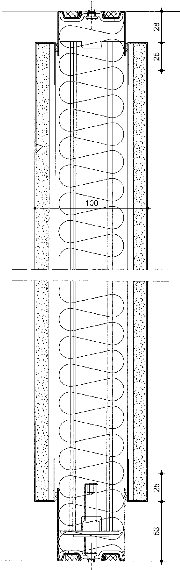
Vollbeplankung M 1:2
