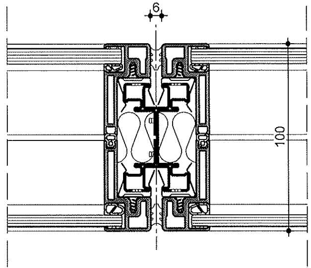
Vollverglasung M 1:2
