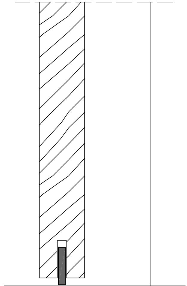
Türzarge M 1:2
