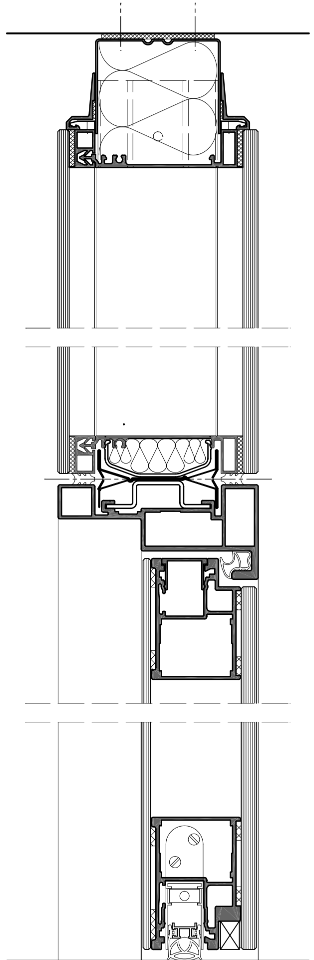
Türelement M 1:2
