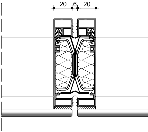
Einscheibenverglasung M 1:2
