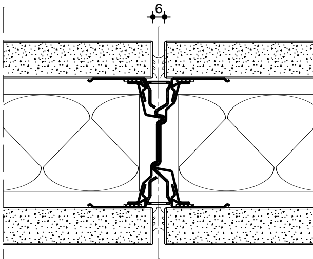
Vollbeplankung mit Regalständer M 1:2
