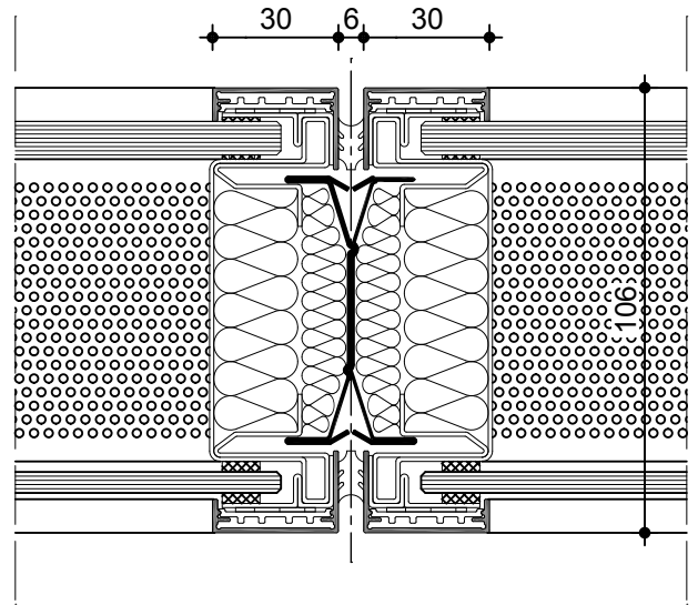
Verglasung M 1:2
