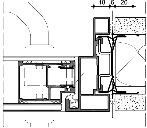
Türzarge/ Vollbeplankung M 1:2
