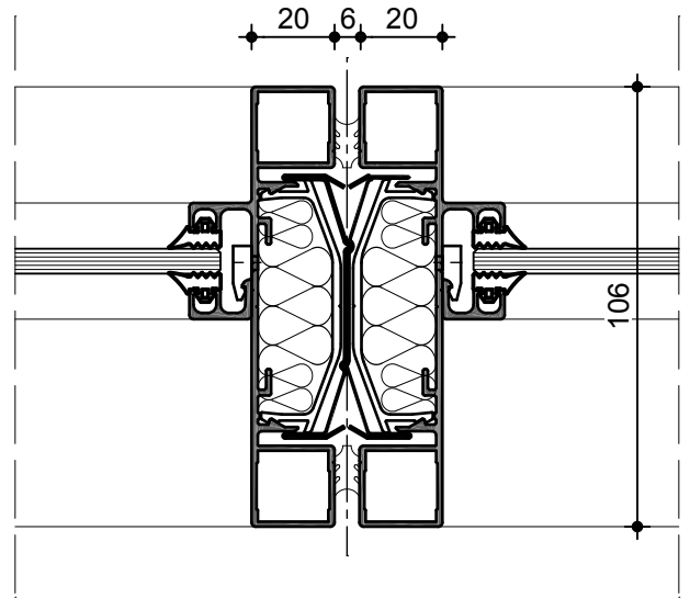
Einscheibenverglasung M 1:2
