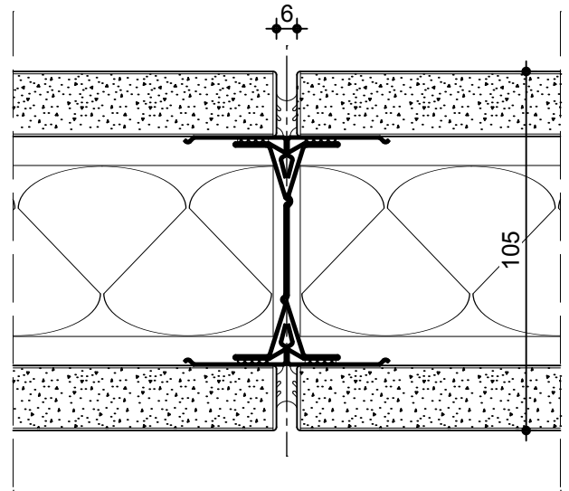
Vollbeplankung M 1:2
