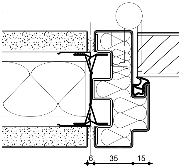
Vollbeplankung / Türzarge M 1:2
