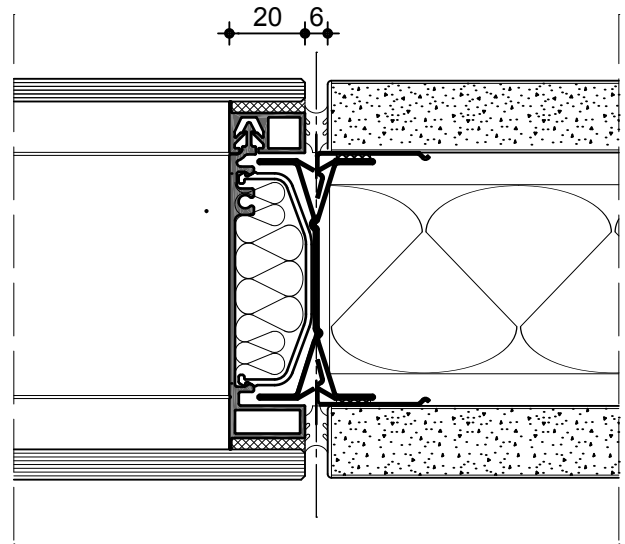
Verglasung / Vollbeplankung M 1:2
