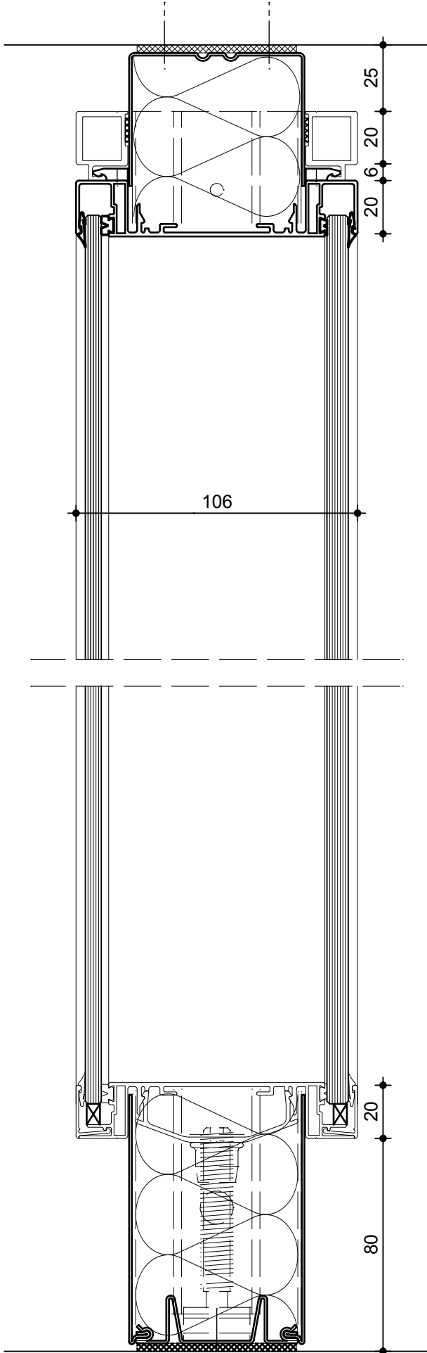
Verglasung M 1:2
