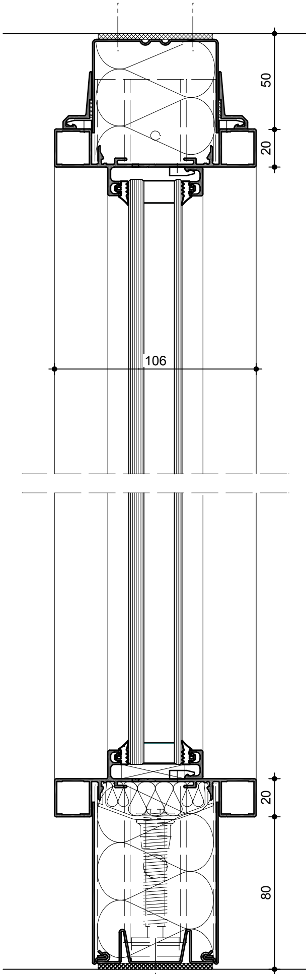
Verglasung Isolierglas M 1:2
