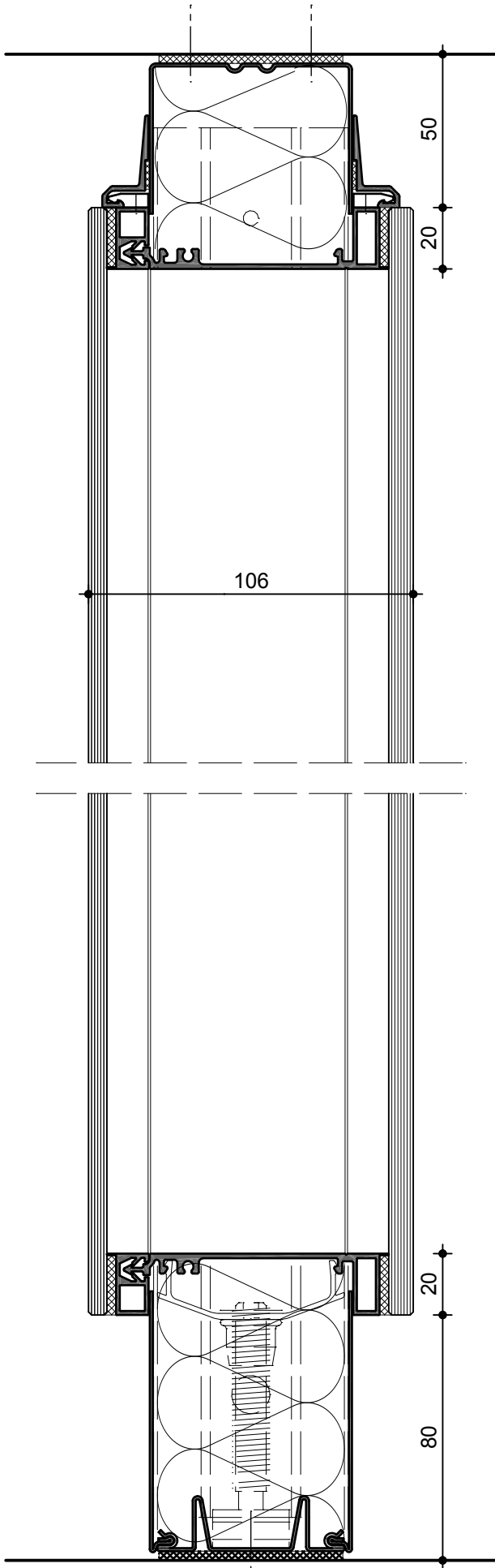
Verglasung M 1:2
