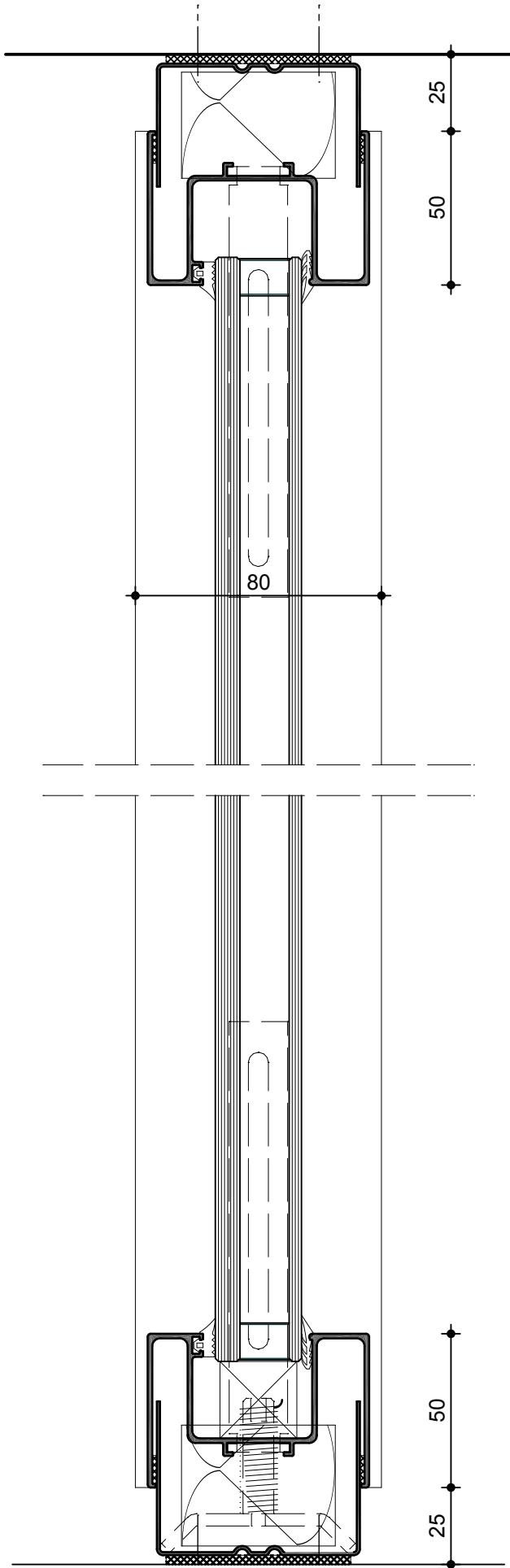
Verglasung Isolierglas M 1:2
