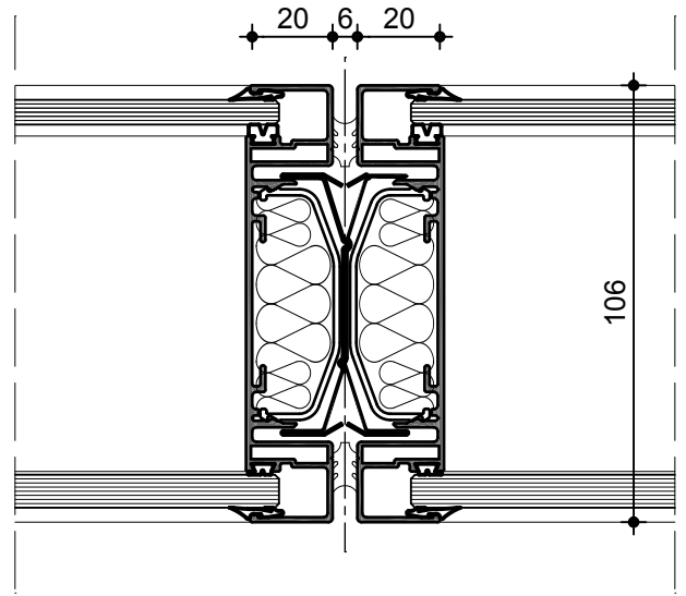
Verglasung M 1:2
