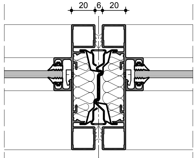
Verglasung mit Regalständer M 1:2
