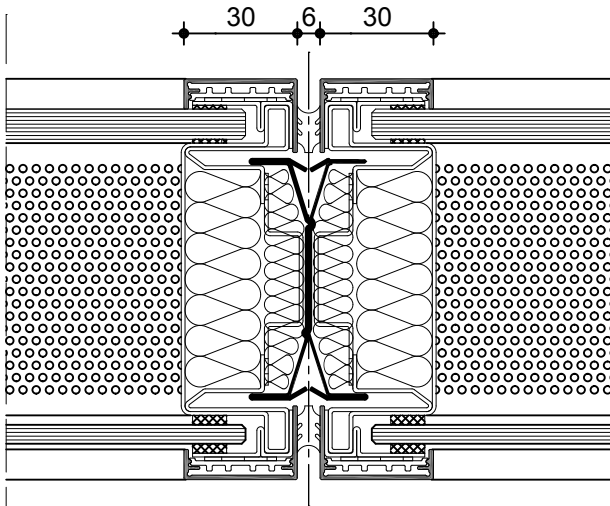
Verglasung EI30 M 1:2
