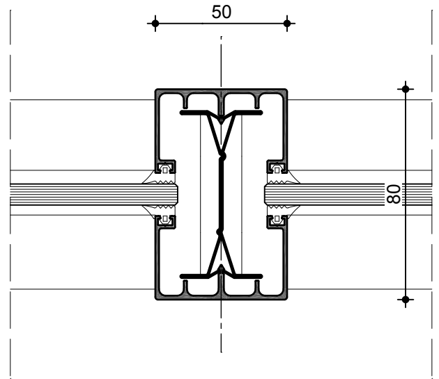
Einscheibenverglasung M 1:2
