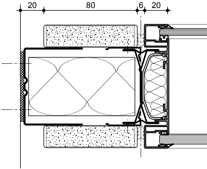
Wandanschluss M 1:2
