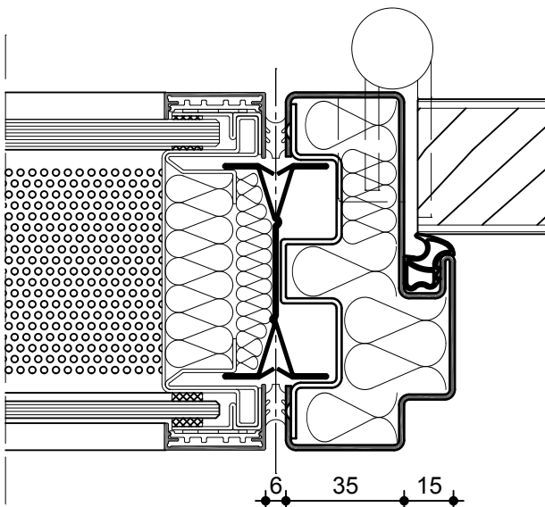
Verglasung / Türzarge M 1:2
