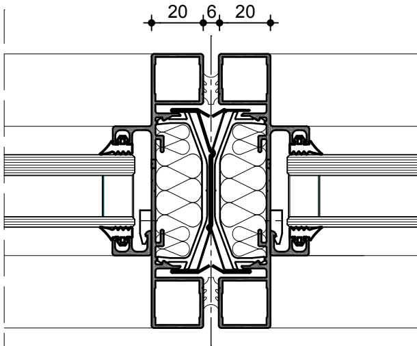
Verglasung Isolierglas M 1:2
