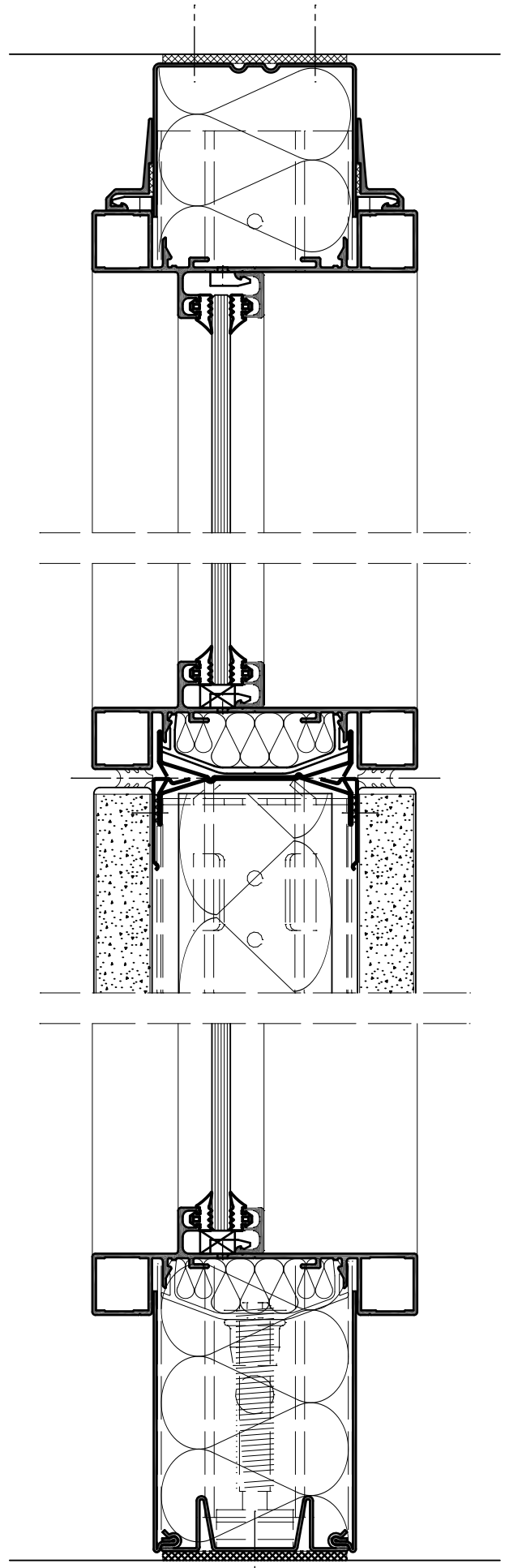
Verglasung M 1:2
