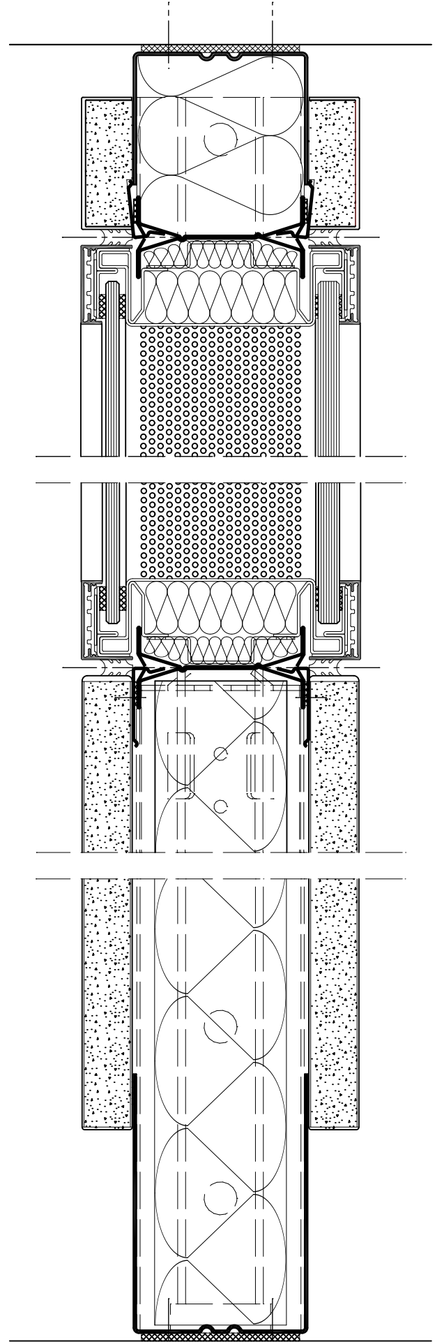
Oblichtverglasung M 1:2
