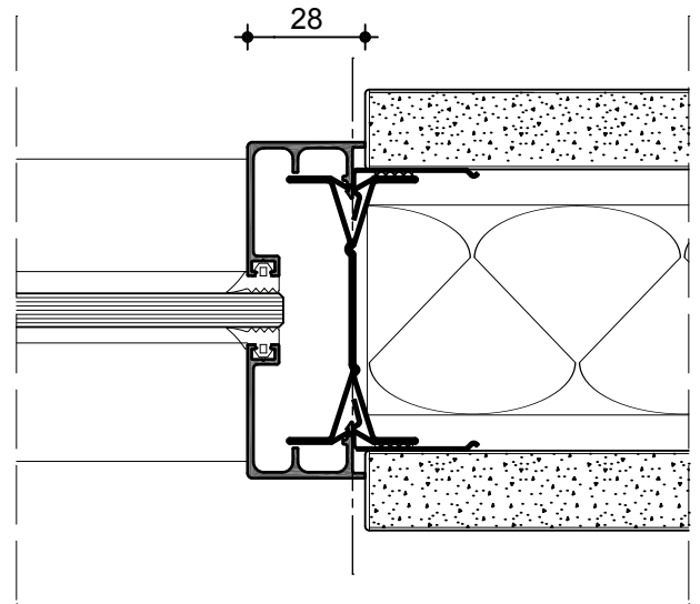
Verglasung / Vollbeplankung M 1:2
