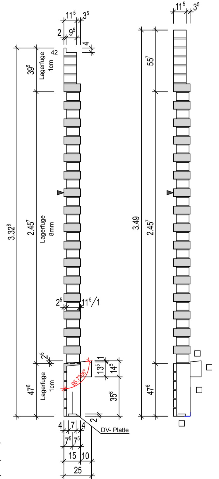
Schnitt B
